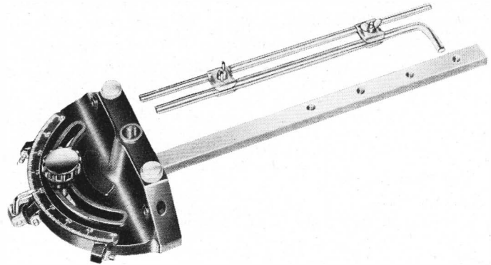
Fig. 18. Auto-Set Miter Gage.
