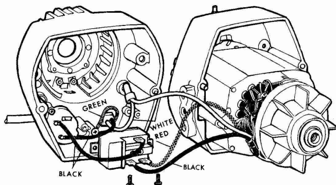
MOTOR WIRING
